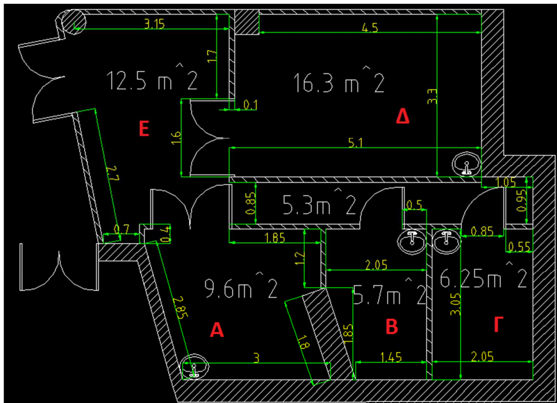
Σχέδιο Α. Τελική διαμόρφωση εργαστηριακών χώρων (κάτοψη)
