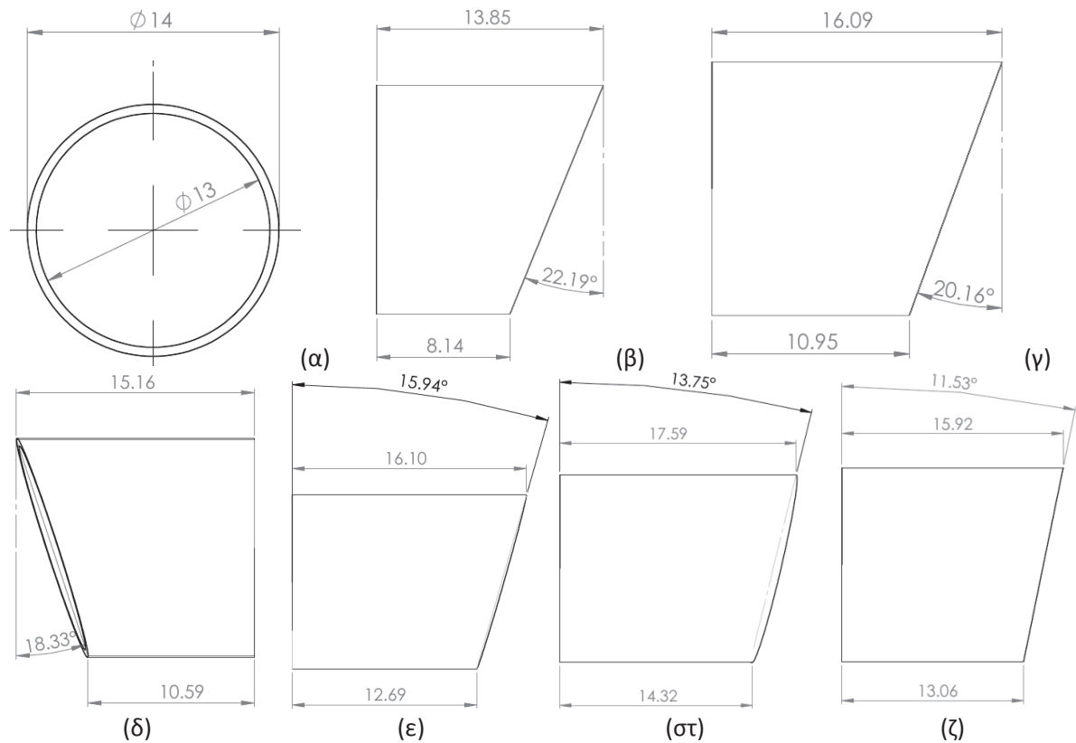
Εικόνα 3. Ενδεικτικές διαστάσεις μεταλλικά νεύρων – γωνιών και θέσεις όπου προβλέπεται να γίνει διάνοιξη σπών με laser (Είδος Β).
