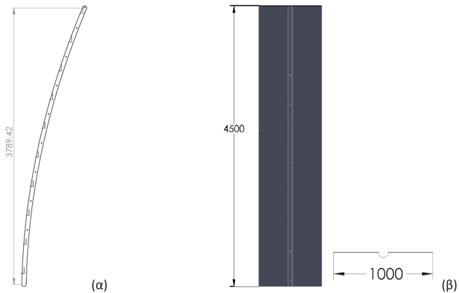
Εικόνα 2. (α) Ενδεικτικές διαστάσεις μεταλλικών ελασμάτων - πλάγιων οδηγών (Είδος A3) και θέσεις όπου προβλέπεται να γίνει χάραξη και διάνοιξη οπών με laser και (β) ενδεικτικές διαστάσεις μεταλλικών ελασμάτων - πτερύγιων (Είδος A4) και θέσεις όπου θα προβλέπεται να γίνουν οπές με χρήση laser.
