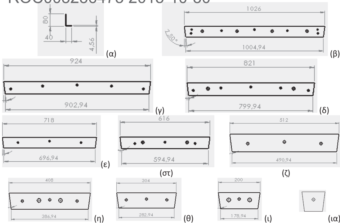
Εικόνα 3. Ενδεικτικές διαστάσεις μεταλλικά νεύρων – γωνιών και θέσεις όπου προβλέπεται να γίνει διάνοιξη σπών με laser (Είδος Β).
