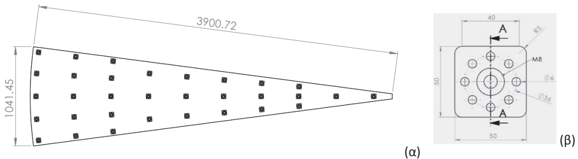
Εικόνα 1. (α) Ενδεικτικές διαστάσεις ελάσματος INOX - πέταλου και θέσεις όπου θα προβλέπεται να γίνει χάραξη με laser (Είδος A1) και (β) ενδεικτικές διαστάσεις ελάσματος INOX – τακάκι (Είδος A2) και θέσεις όπου θα προβλέπεται να γίνουν οπές με χρήση laser.
