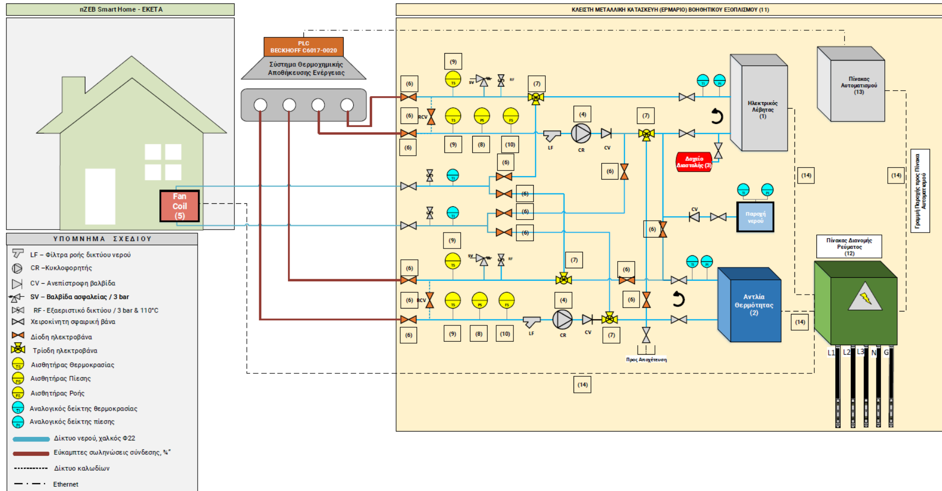
Σχήμα 1: Σχηματική αναπαράσταση της εγκατάστασης του υπό προμήθεια εξοπλισμού
