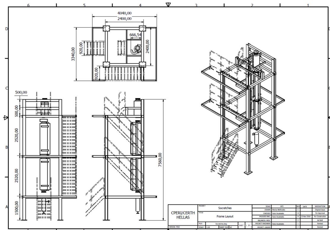
Σχήμα Α.2. Σκαρίφημα συστήματος δύο διαστάσεων
