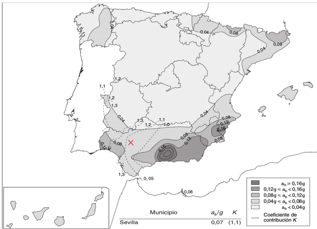
Σχήμα Α.9. Σεισμικός χάρτης κινδύνου Ισπανία και συντελεστής σεισμικότητας για την Σεβίλλη
