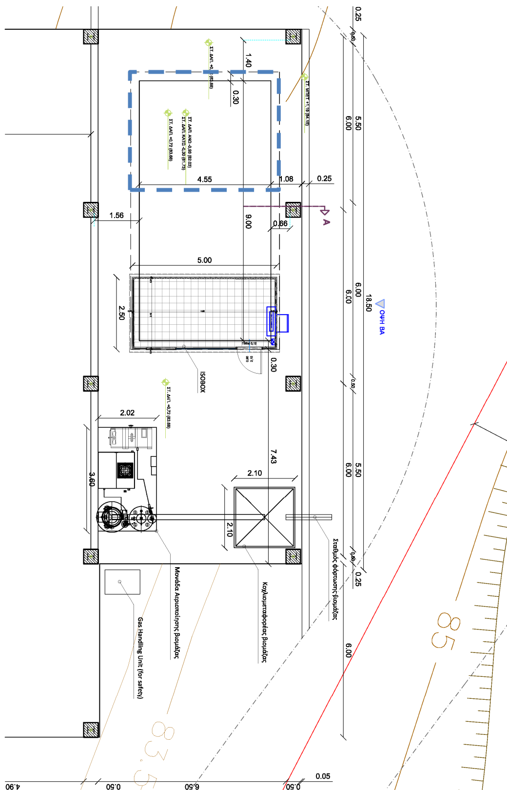
Σχήμα Α.1. Κάτοψη περιοχής έδρασης της μονάδας SOCRATCES. Θέση έδρασης εντός του μπλε πλαισίου.
