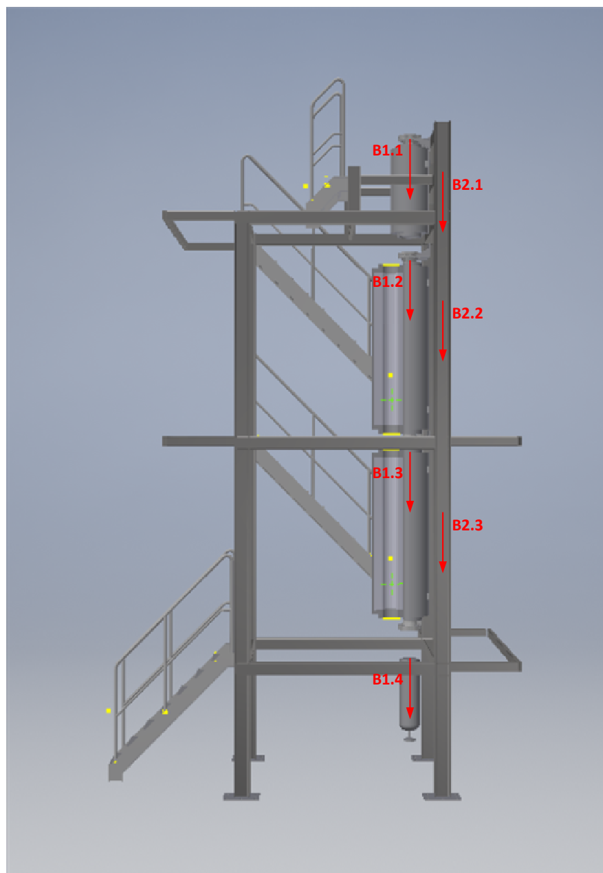
Σχήμα Α.3. Απεικόνιση σίδηρο-κατασκευής, αντιδραστήρων, δοχείων και φούρνων και τα επιμέρους βάρη τους
