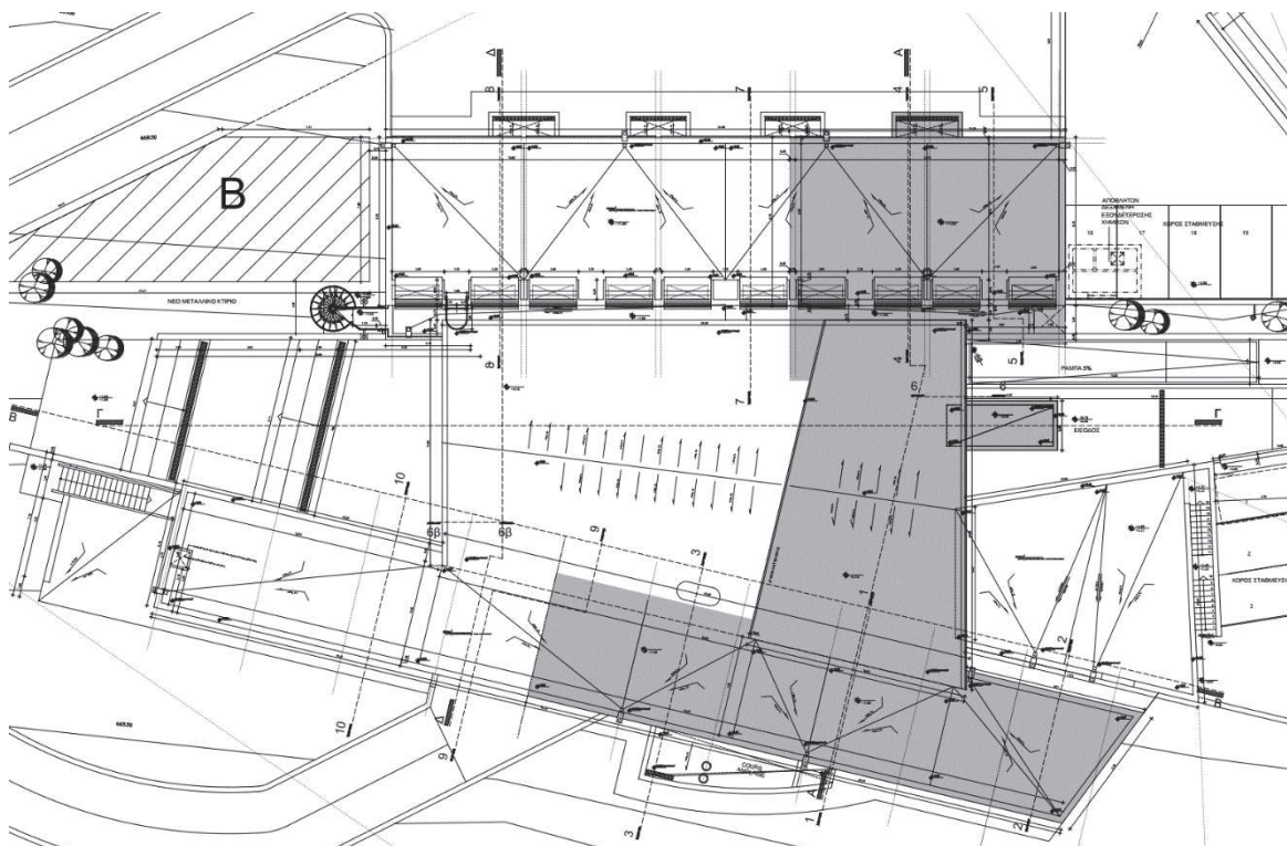
Εικόνα 1: Κάτοψη οροφής υφιστάμενου κτιρίου (σκιασμένη επιφάνεια) και επέκτασης
