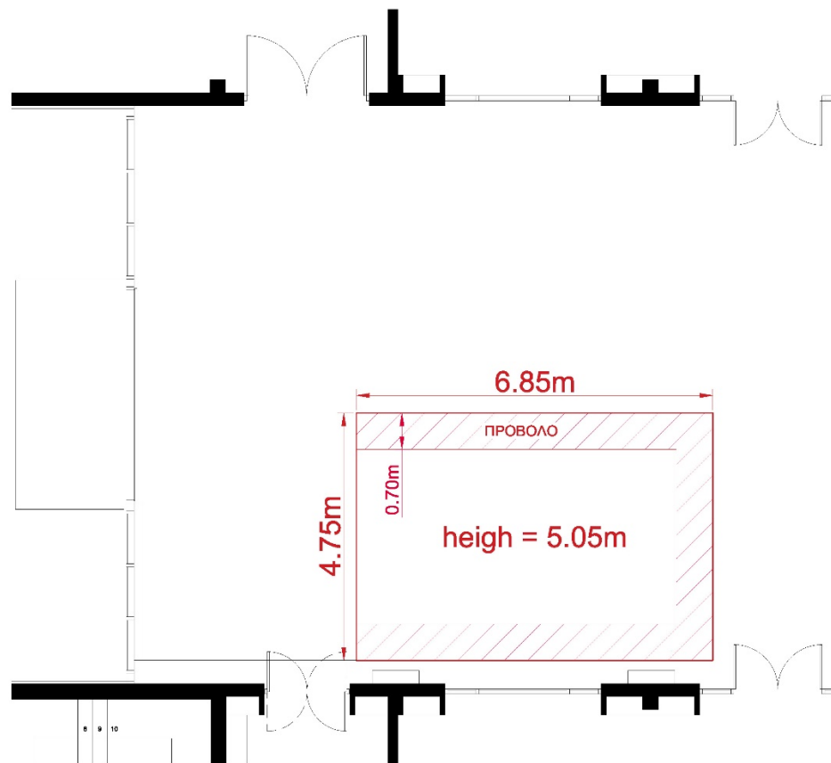
Σχήμα Α.1. Κάτοψη περιοχής έδρασης της μεταλλικής κατασκευής. Θέση έδρασης εντός του κόκκινου πλαισίου.
